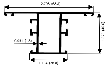
DIVISOR INTERMEDIO
