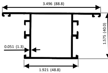
DIVISOR INTERMEDIO
